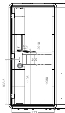
4 Power module
